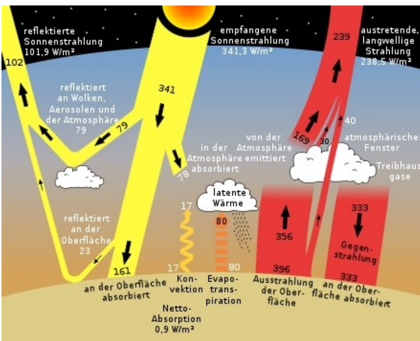
1 Die Energiebilanz der Erde
